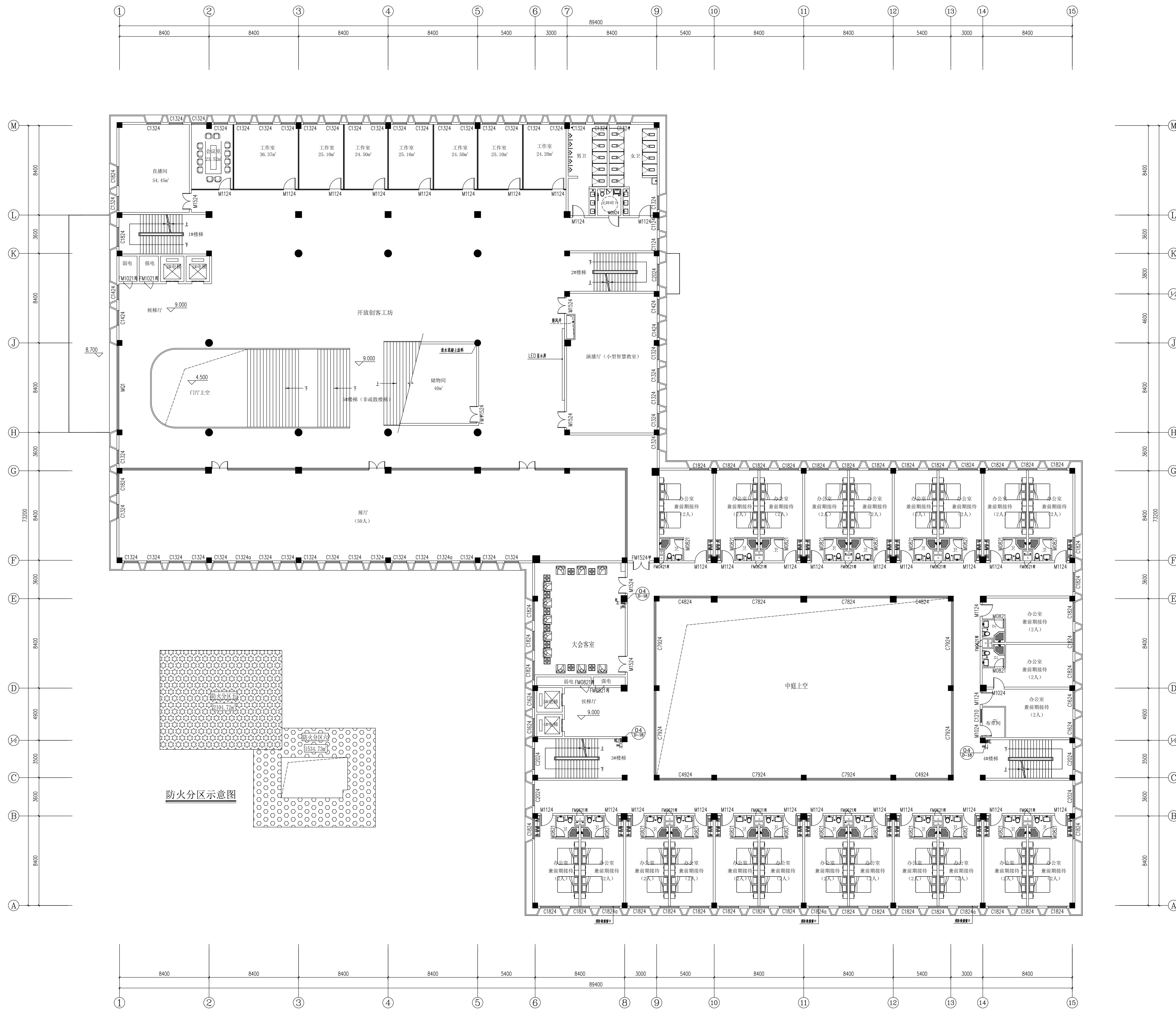
三层平面及索引图 1:125
